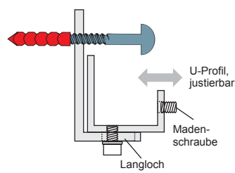
unteres Befestigungselement
