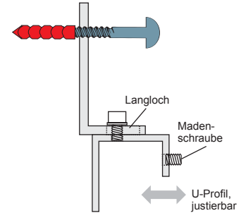
oberes Befestigungselement
